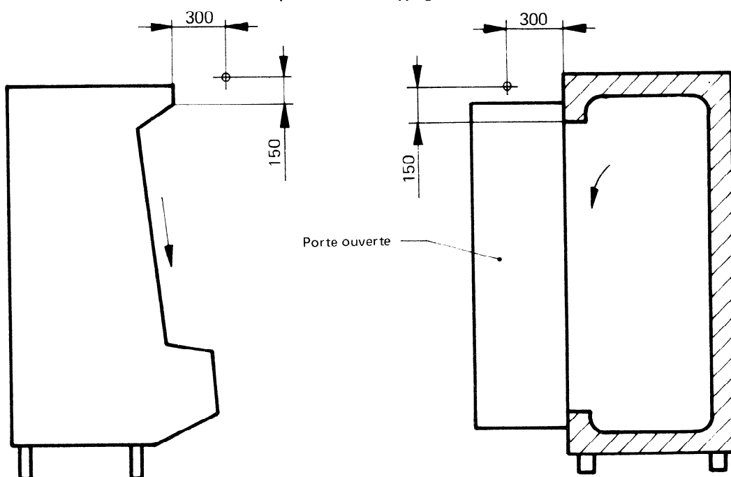
FIGURE 4 – Point de mesurage de l'ambiance pour meubles de type vertical
