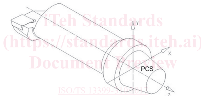
Figure 4 — Position de l'outil rond — Plan de jauge ou surface de contact planeaire
