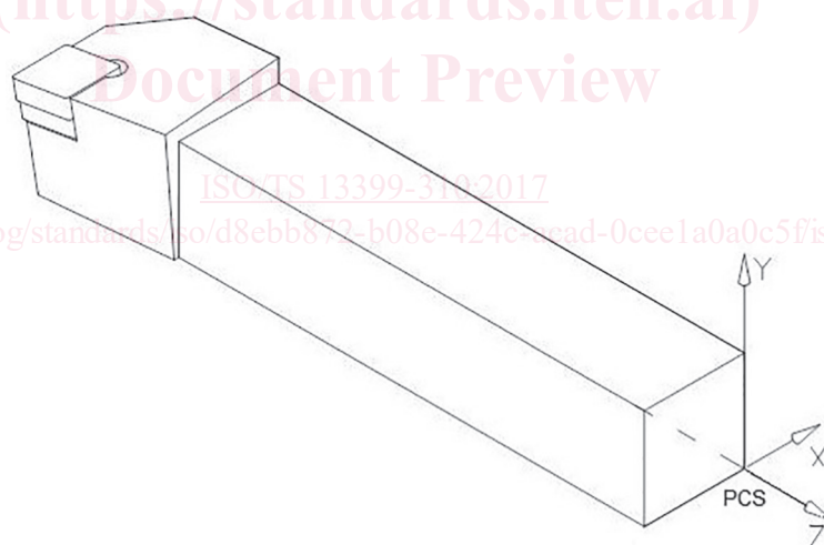
Figure 2 — Position de l'outil prismatique
