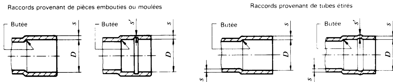
Figure 3 — Épaisseur de paroi
