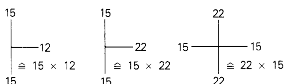
Figure 6 — Désignation des tés et croix de diamètre égal le long du passage et de diamètre réduit ou élargi sur l'embranchement ou de diamètre symétriquement réduit sur les embranchements
