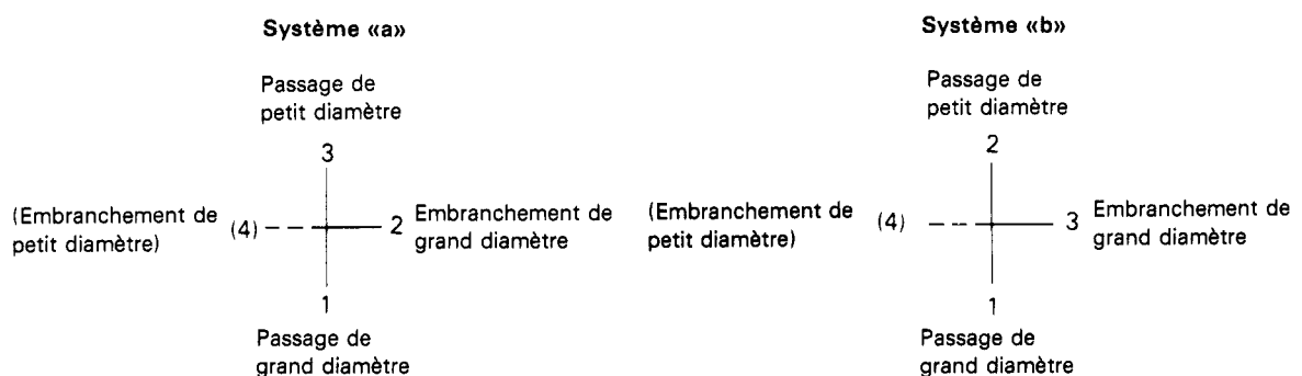
Figure 5 — Désignation des té (et croix)
