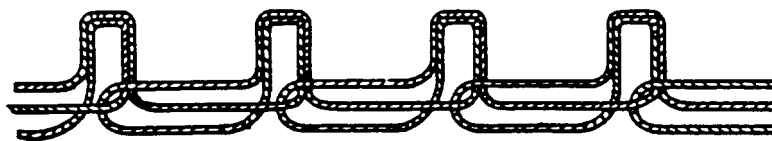
FIG. 4 Stitch Type 104
