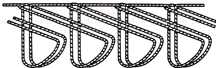
FIG. 3 Stitch Type 103
