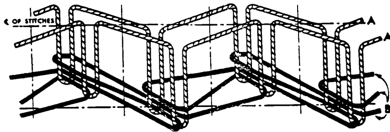
FIG. 31 Stitch Type 405
