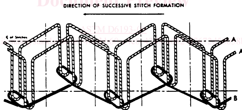
FIG. 14 Stitch Type 304
