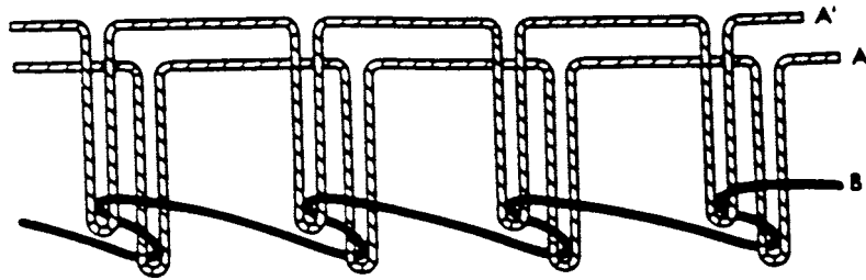
FIG. 19 Stitch Type 309
