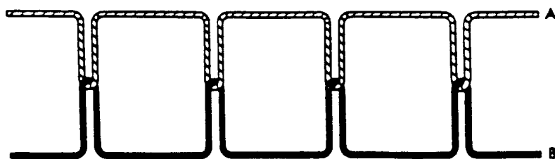
FIG. 10 Stitch Type 205
