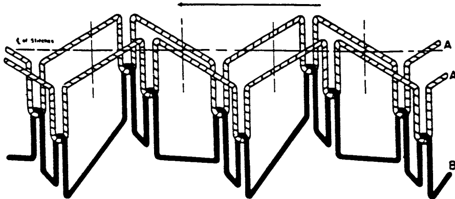
FIG. 22 Stitch Type 312
