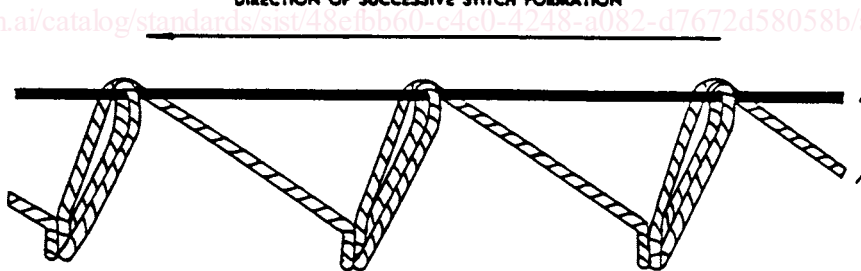
FIG. 23 Stitch Type 313
