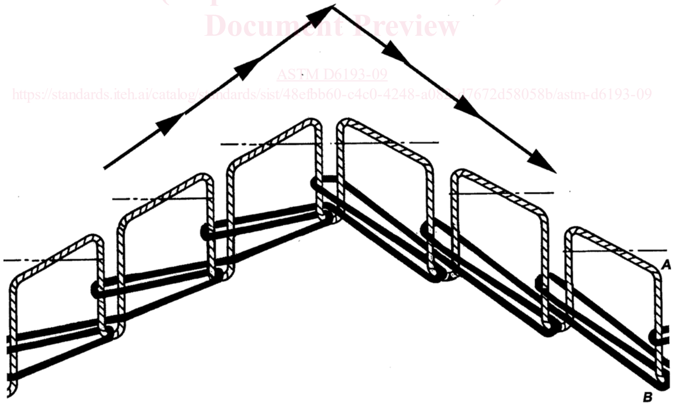
FIG. 34 Stitch Type 408
