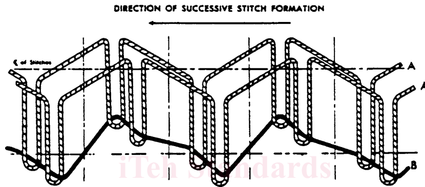
FIG. 19 Stitch Type 309
