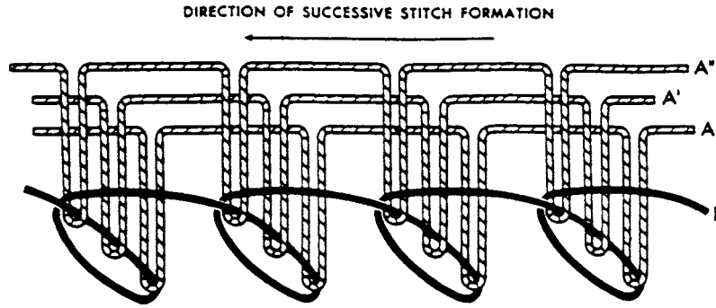
FIG. 13 Stitch Type 303
