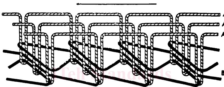
FIG. 28 Stitch Type 402
