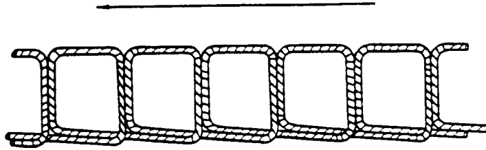
FIG. 7 Stitch Type 202
