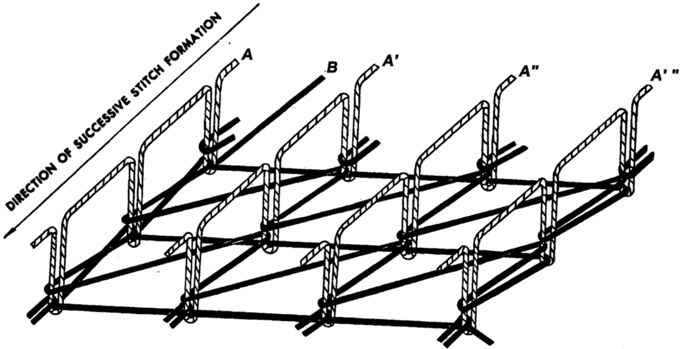
FIG. 34 Stitch Type 408
