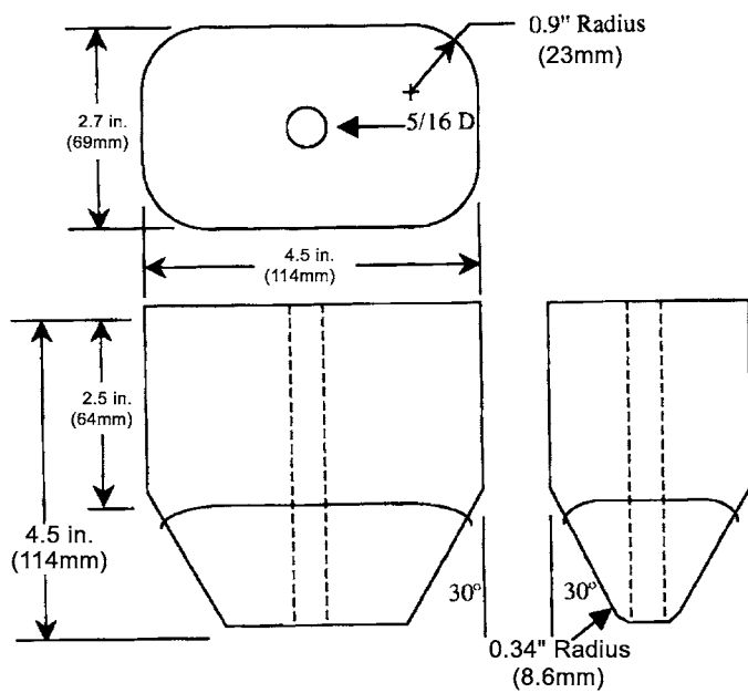
FIG. 2 Torso Probe
