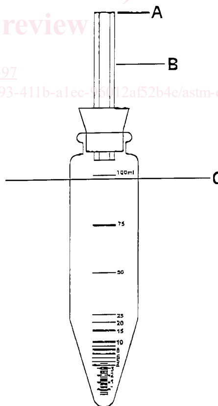
FIG. 1 Apparatus Assembly
