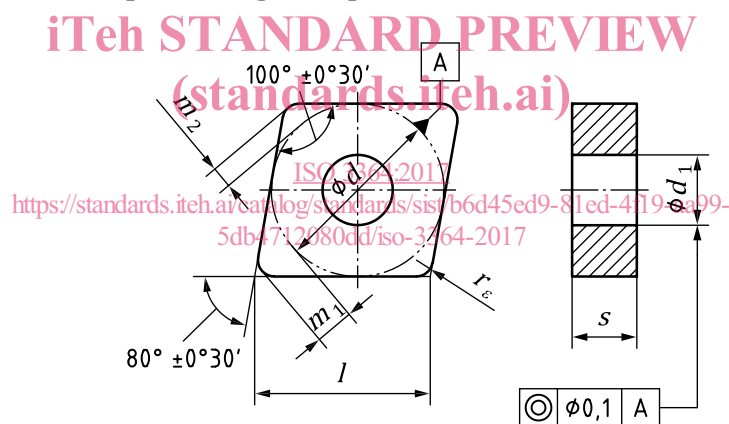
a) CN.A sans brise-copeaux
