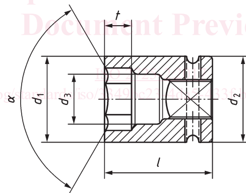
Figure 1 — Douilles avec d_1 < d_2
