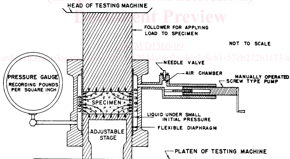
FIG. 1 Hveem Stabilometer
