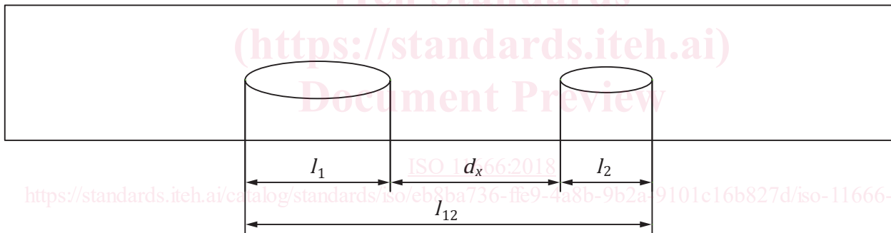
Figure 1 — Configuration géométrique pour les discontinuités groupées
