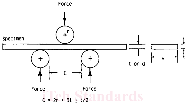
FIG. 2 Transverse Bend Test
