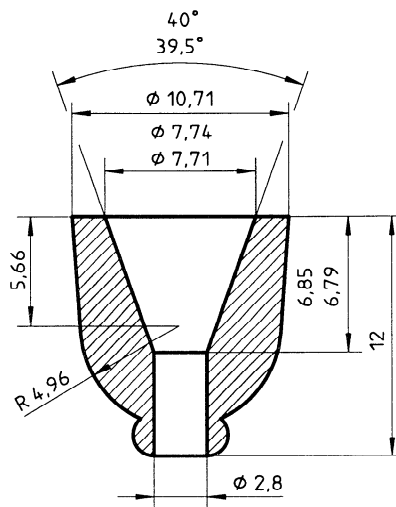
Figure 4 — Jauge de profondeur pour thermomètre
