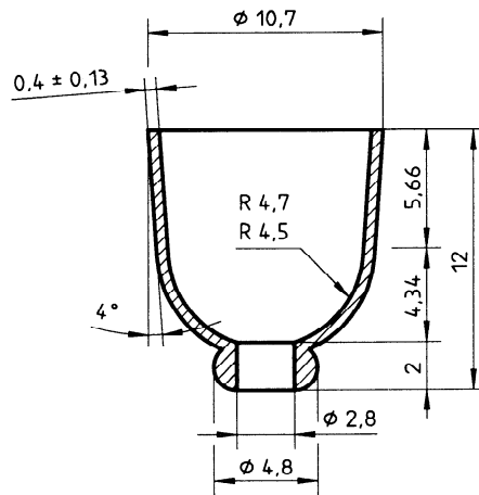
Figure 1 — Coupelle à graisse
