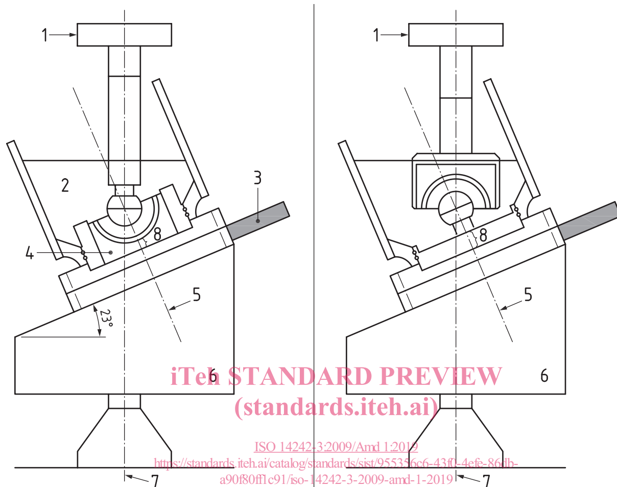
a) Position inversée (parfois utilisée pour les essais d'usure comprenant des particules de troisième corps)
