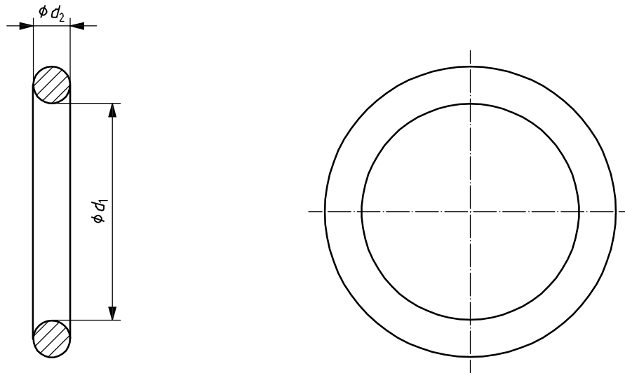
Figure 1 — Configuration type d'un joint torique (standards.iteh.ai)
