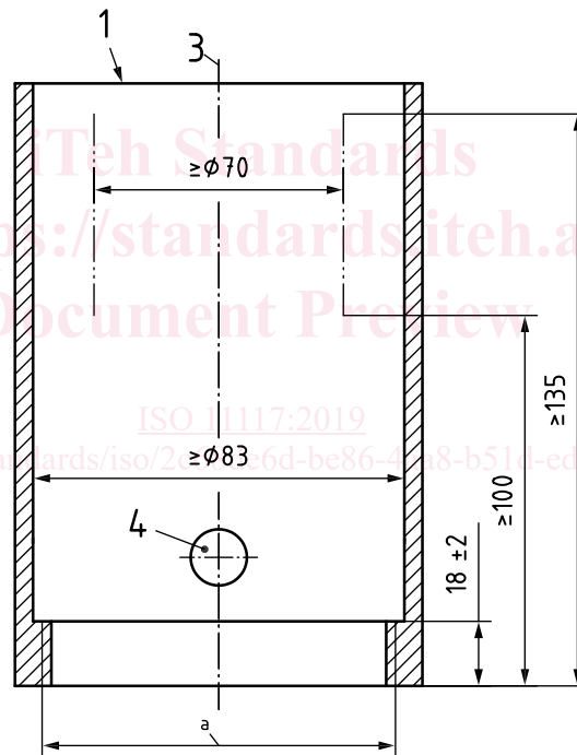
a) Chapeau fermé découvert de protection de robinet
