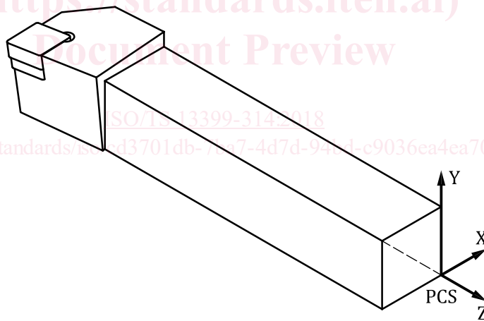
Figure 2 — Position de l'outil prismatique
