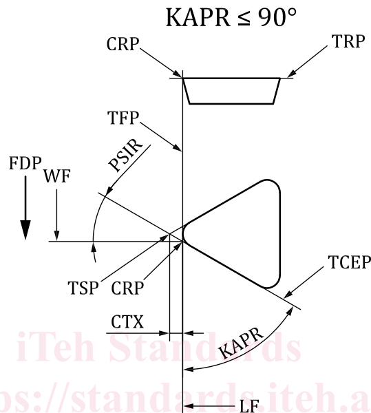
Figure 4 — Direction d'avance perpendiculaire à l'axe de l'outil — KAPR \leq 90^\circ
