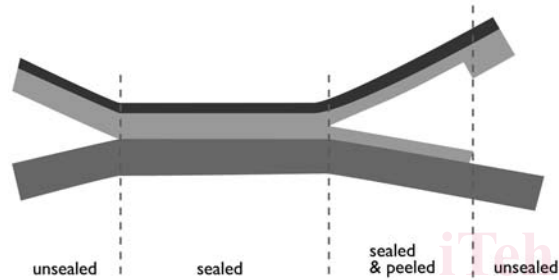
COHESIVE PEEL
