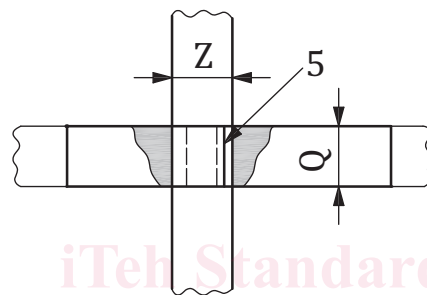
a) joint normal bout-à-bout de raboutage
