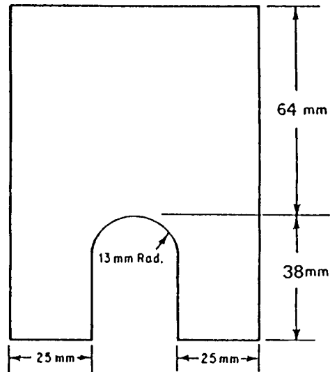
FIG. 1 Keel Block for Test Coupons
