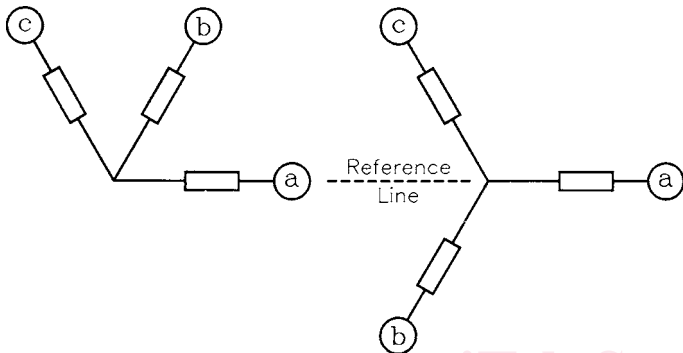
FIG. 2 0° – 60° – 120° Rosette
