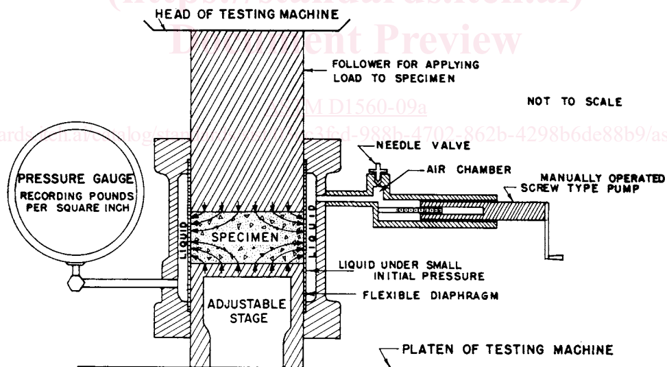
FIG. 1 Hveem Stabilometer
