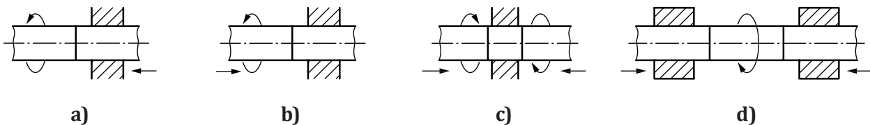
Figure 5 — Méthodes de soudage par friction rotative
