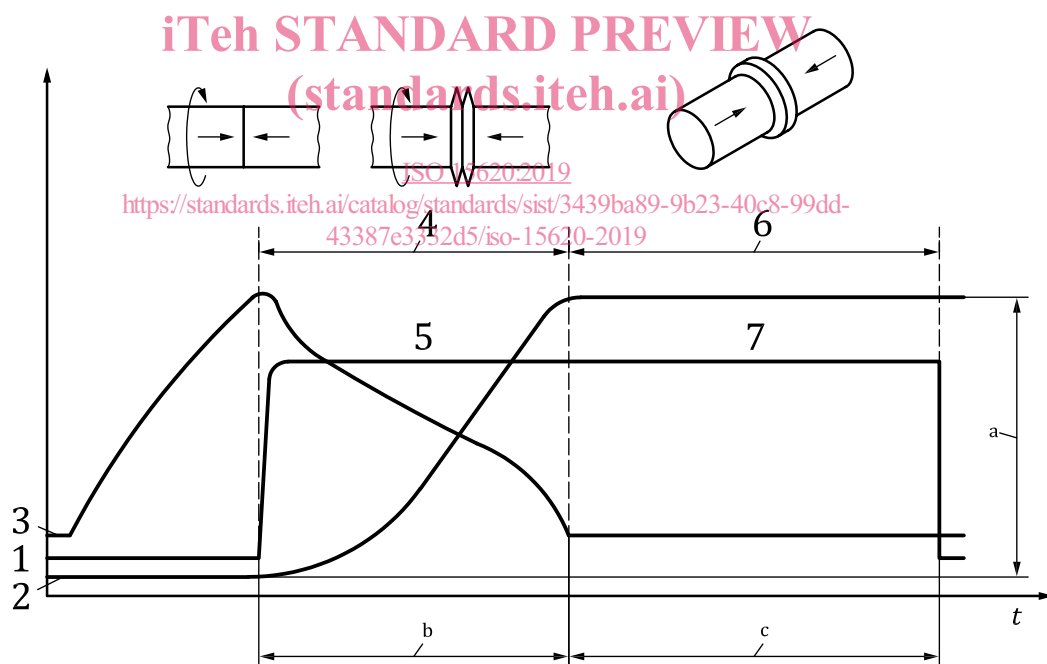
Figure 3 — Schéma du soudage par friction par inertie
