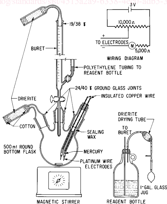
FIG. 1 Titration Assembly
