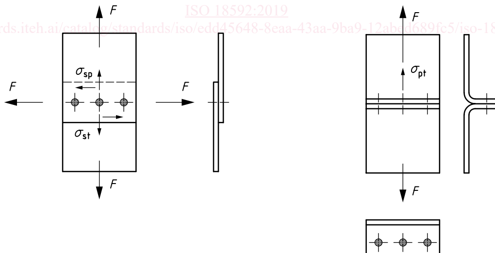
a) Effort de cisaillement transversal à la ligne de joint et effort de cisaillement parallèle dans l'axe de la ligne de joint
