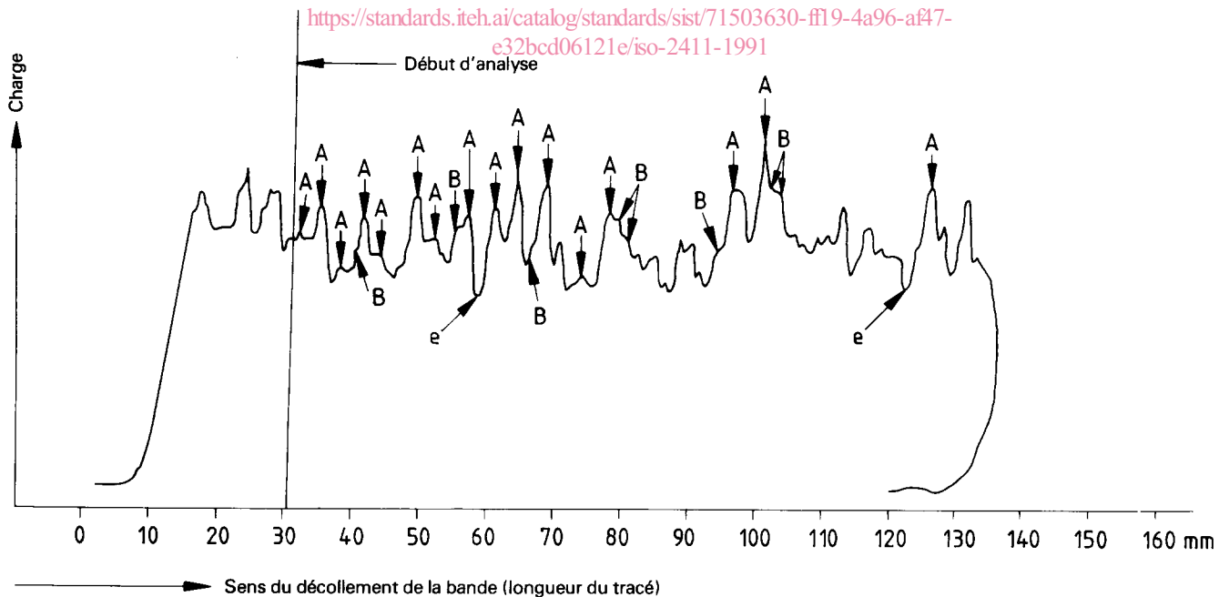
b) Réponse mécanique en cas de faible inertie
