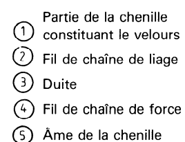
Figure 7 — Moquette chenille «Axminster» (coupe dans le sens chaîne)
