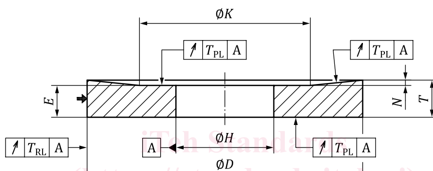
Figure 6 — Meule à dépouille sur un côté (Type 20)
