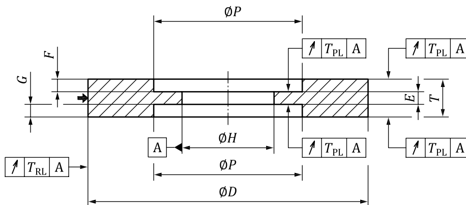
Figure 5 — Meule à deux embrèvements (Type 7)
