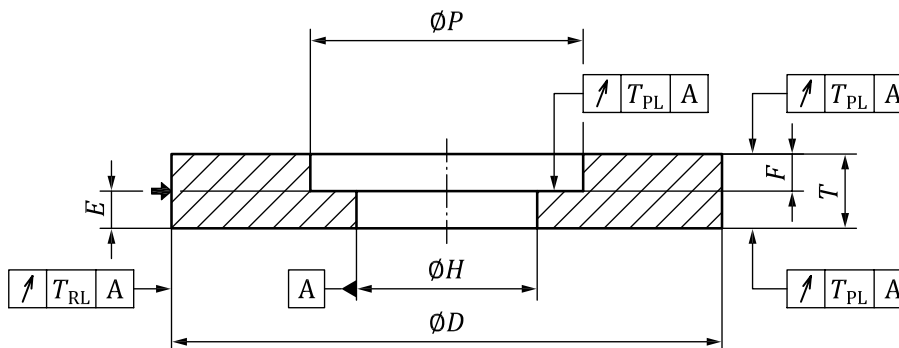
Figure 4 — Meule à un embrèvement (Type 5)
