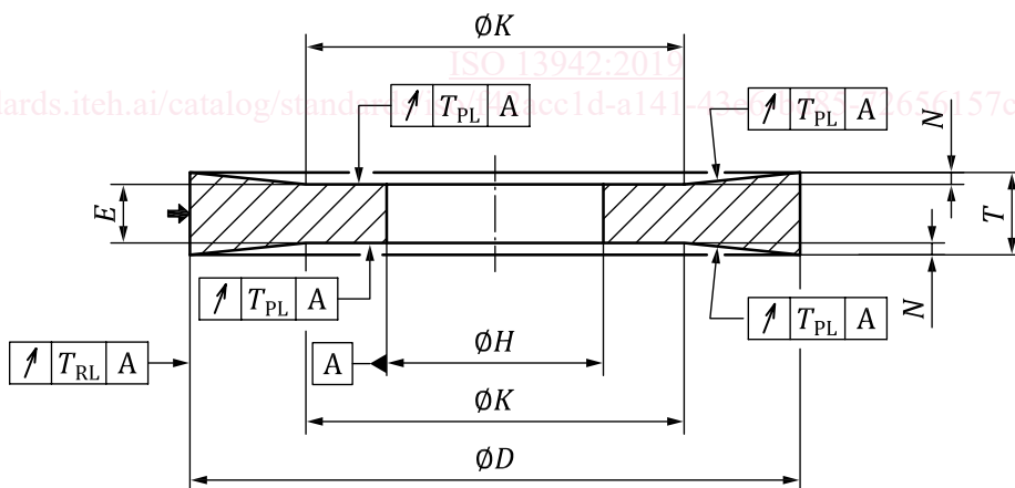
Figure 7 — Meule à dépouille sur deux côtés (Type 21)
