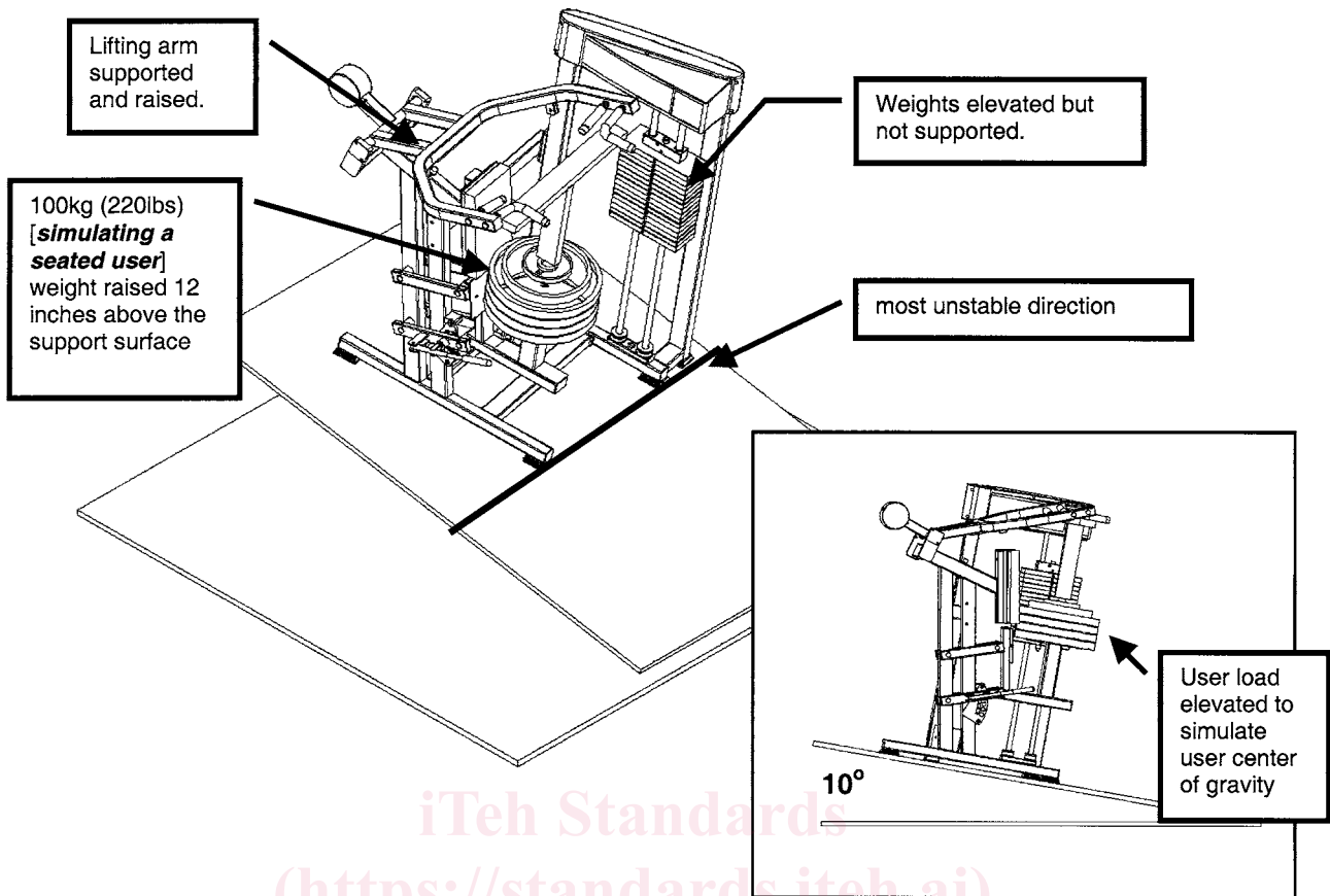
FIG. 1 Tilt Test
