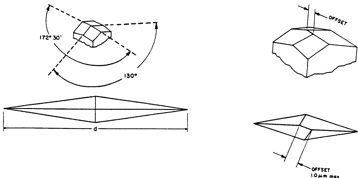
FIG. 2 Knoop Indenter
