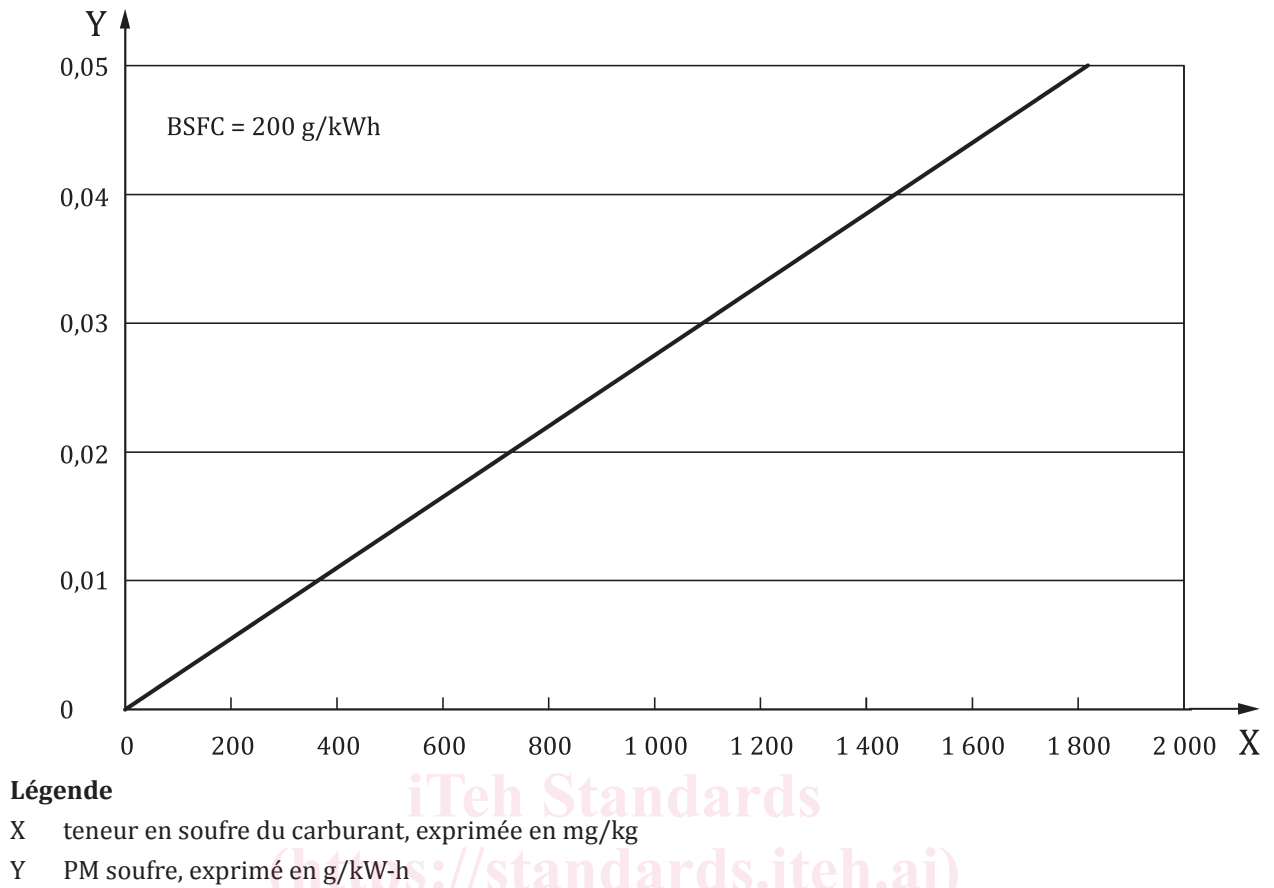
Figure 1 — Relation entre la teneur en soufre du carburant et l'émission de sulfates pour des moteurs sans traitement postcombustion des gaz d'échappement
