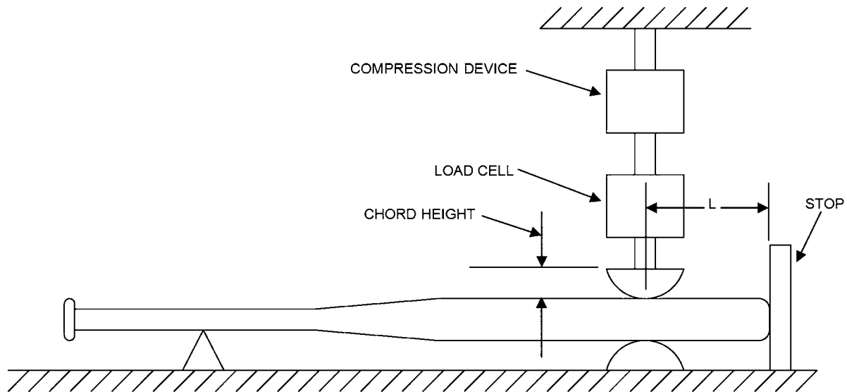
FIG. 1 Test Apparatus
