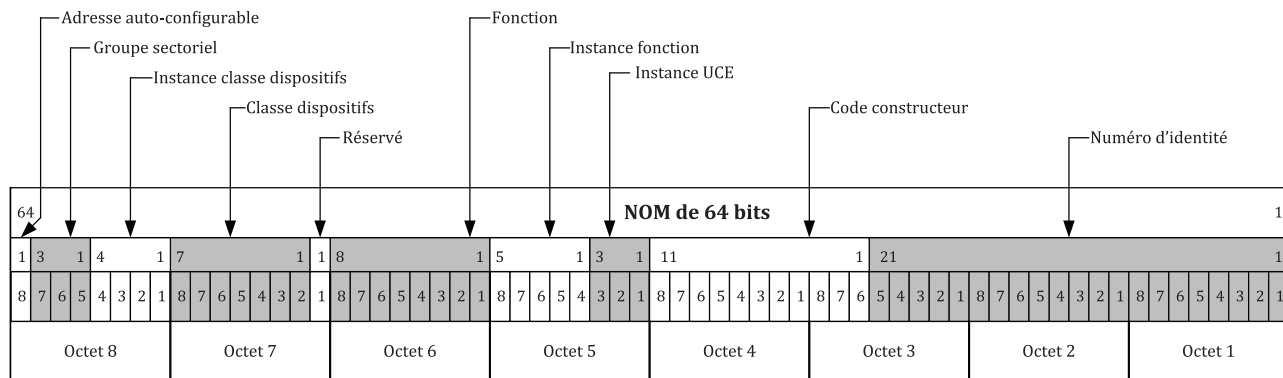
Figure 1 — Champs des bits NOM dans les octets de données d'un message CAN
