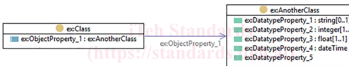
Figure 1 — Notation UML pour les classes et les propriétés
