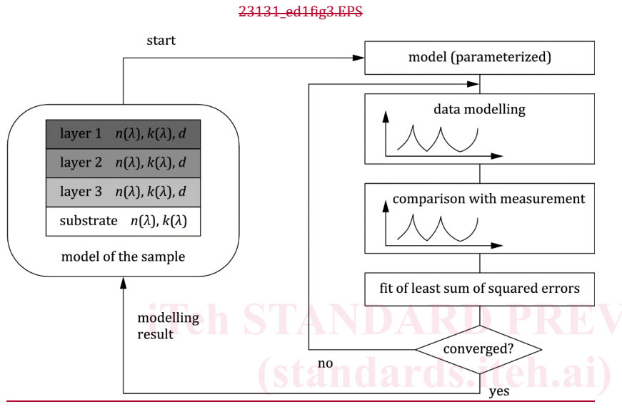
Figure 3 — Représentation schématique de la procédure de régression itérative
