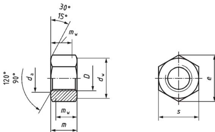
Figure 1 — Ecrou sans collerette au niveau de la face d'appui
