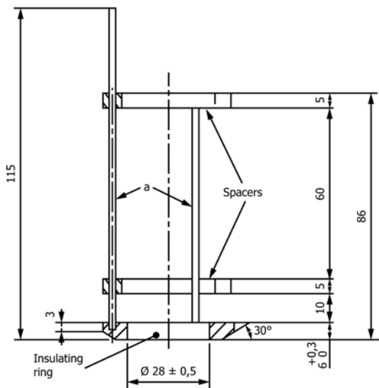
FIG. 3 Spacers
