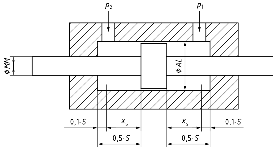
Figure 1 — Identification d'un vérin double tige
