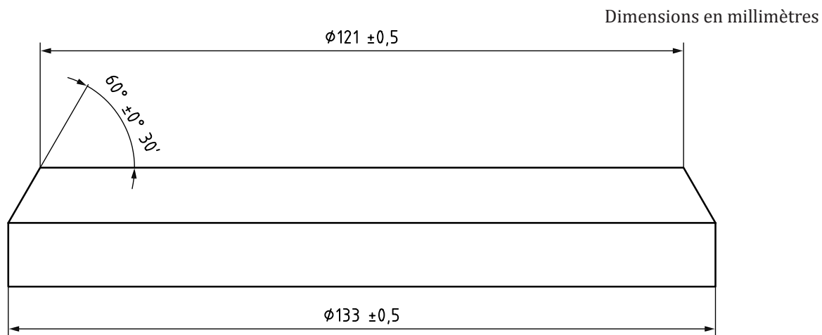
Figure 1 — Plateau à boulochage iTeh STANDARD PREVIEW (standards.iteh.ai)
