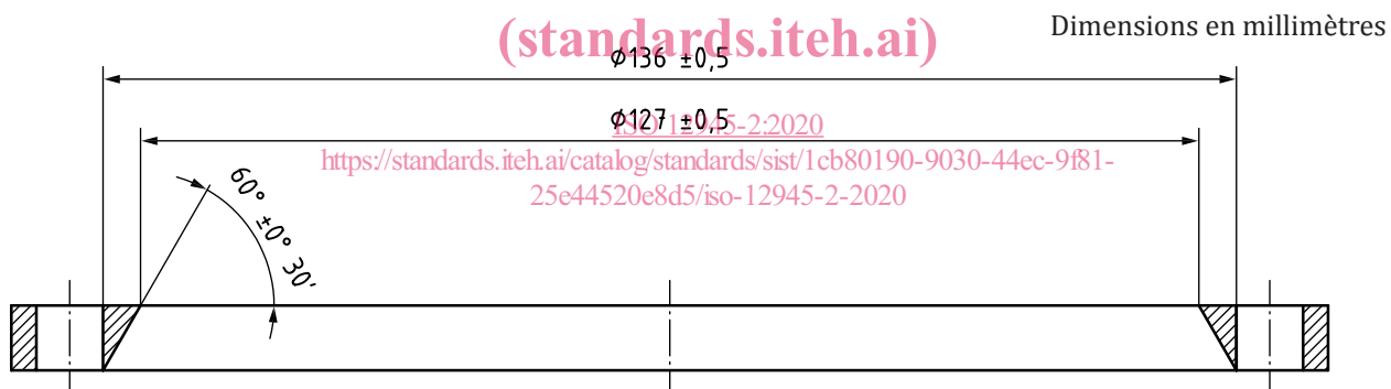
Figure 2 — Anneau de fixation
