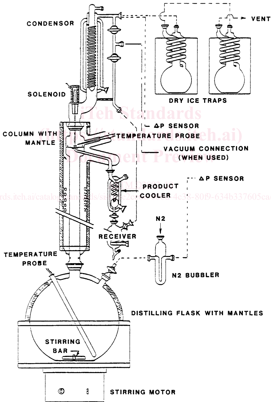
FIG. 1 Apparatus
