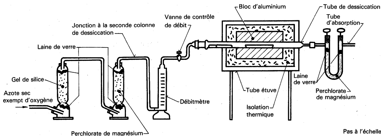
Figure 1 — Appareillage pour la détermination de l'humidité hygroscopique — Méthode 1 (méthode gravimétrique)
