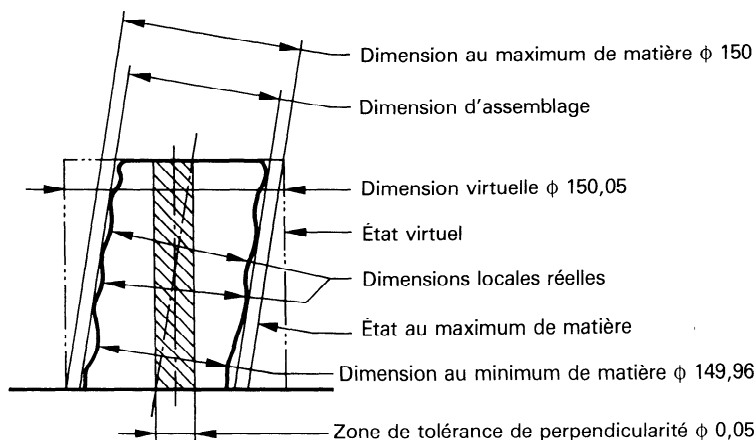
b) Cotation selon le principe de l'enveloppe
