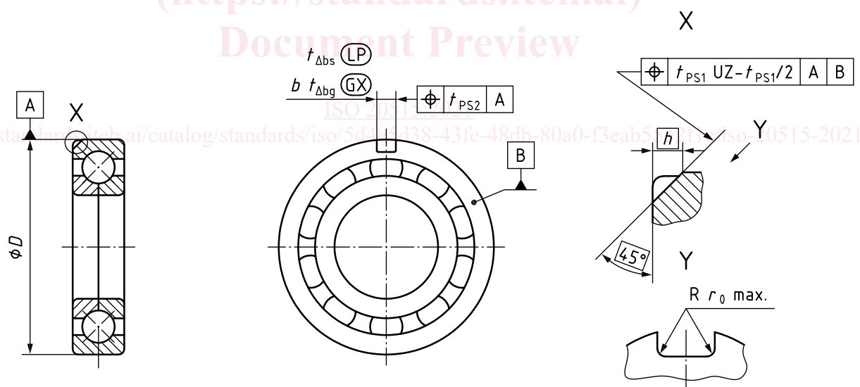
Figure 1 — Roulement radial avec une encoche de retenue
