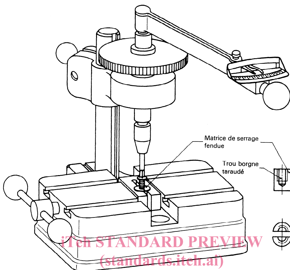
ISO 2702:1992 Figure 1 — Dispositif d'essai à la torsion https://standards.iteh.ai/catalog/standards/sist/bd845f24-70c5-4025-9fc2-ac28074446aa/iso-2702-1992
