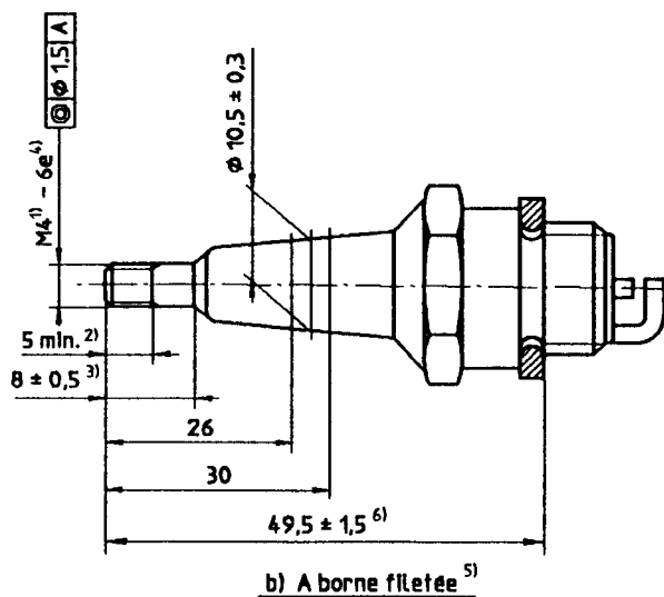
Figure 1 — Bougie d'allumage M12 × 1,25 à siège plat
