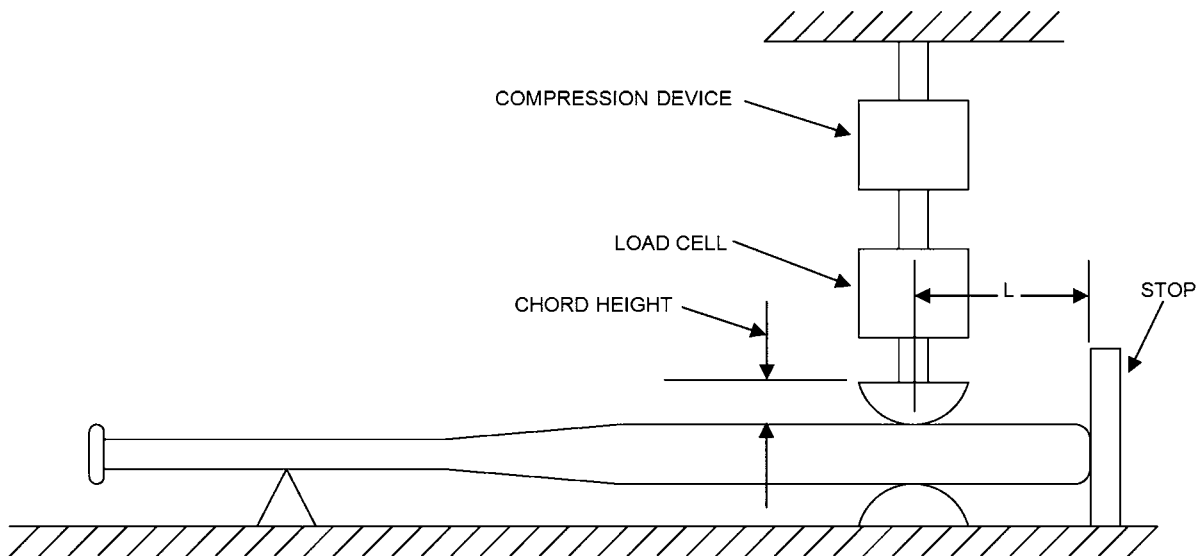
FIG. 1 Test Apparatus
