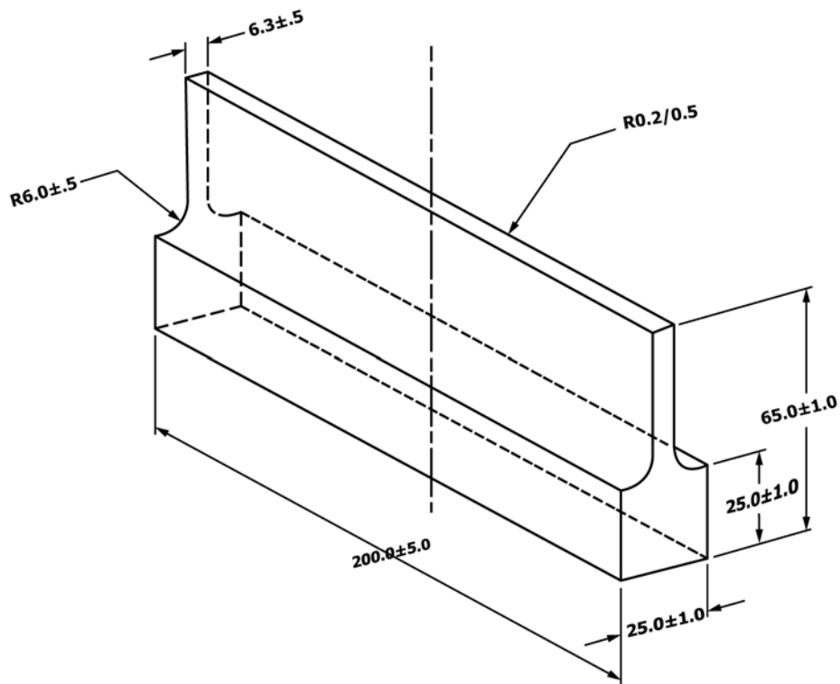
FIG. 1 Edge Anvil
