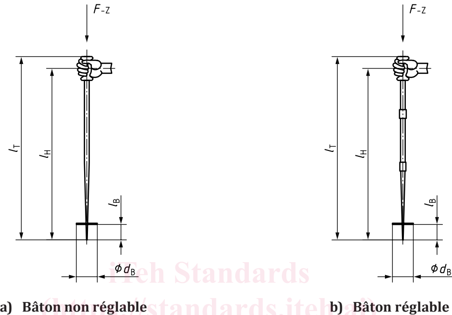
Figure 2 — Centre de rotation et dimensions d'un bâton de ski
