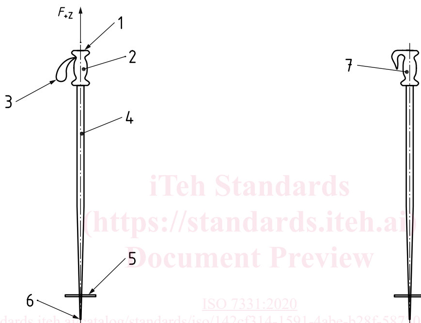
a) Bâton de ski muni d'une poignée avec dragonne
