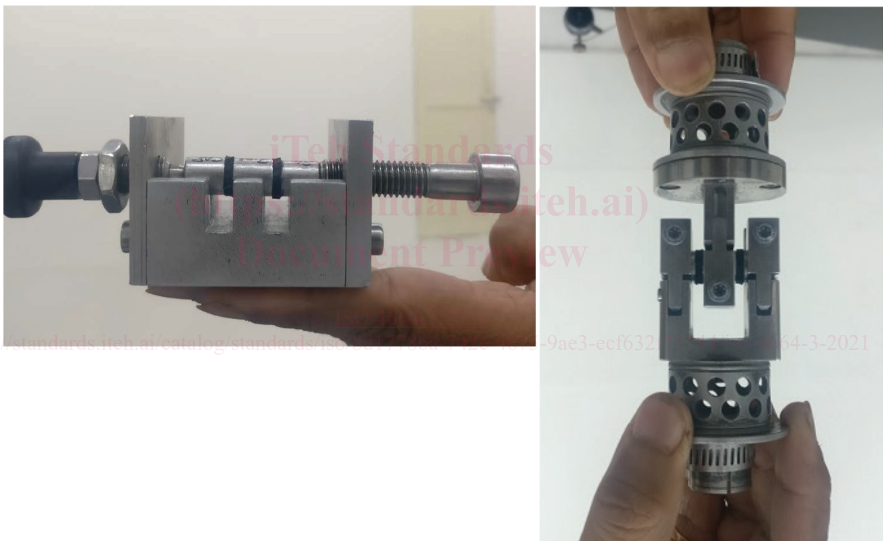
Figure 1 — Exemple d'outil de préparation de l'échantillon de cisaillement et mâchoire correspondante
