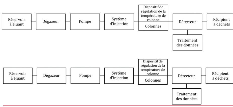
Figure 1 — Schéma d'un appareillage de GPC
